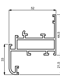
6 Profilo vz.1530
