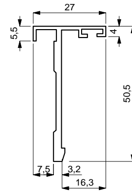
Profilo Mod. 1750
