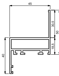
3 Profilo vz.1477
