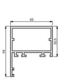
5 Profilo vz.1448
