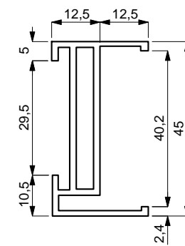
Profilo Mod. 1755
