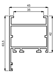
4 Profilo vz.1588
