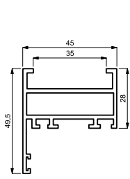
2 Profilo vz.1556
