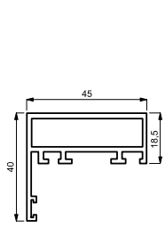
1 Profilo vz.1550
