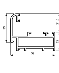
7 Profilo vz.1530
